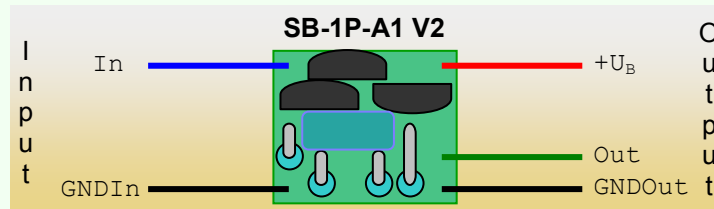
Abbildung 3-1: Die Platine des SB-1P-A1
