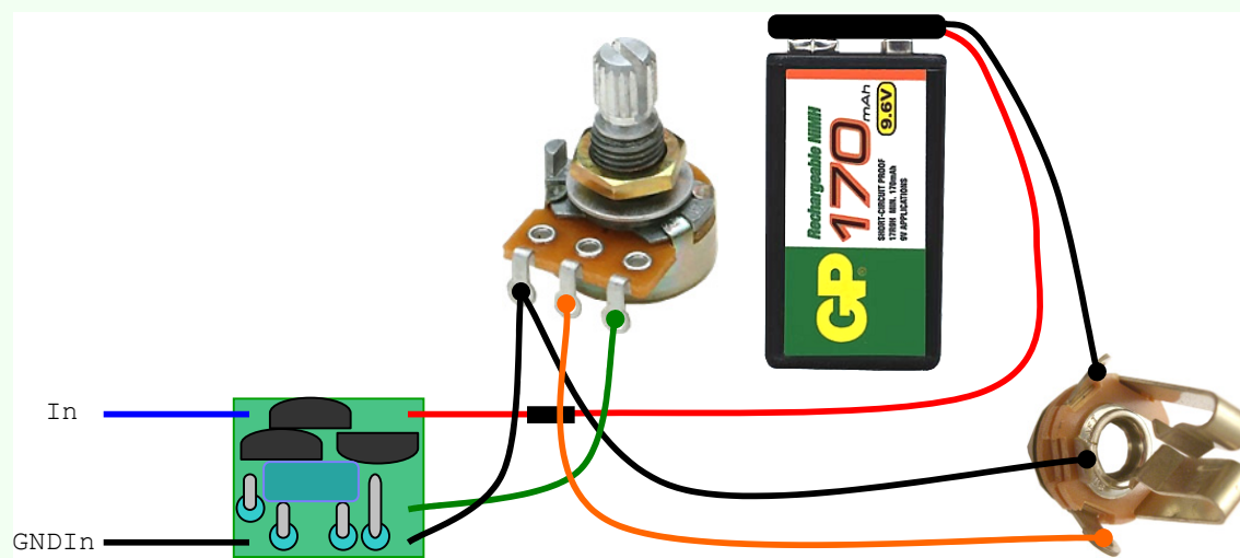
Abbildung 3-3: SB-1P-A1 mit Lautstärkeinsteller vor der Ausgangsbuchse
