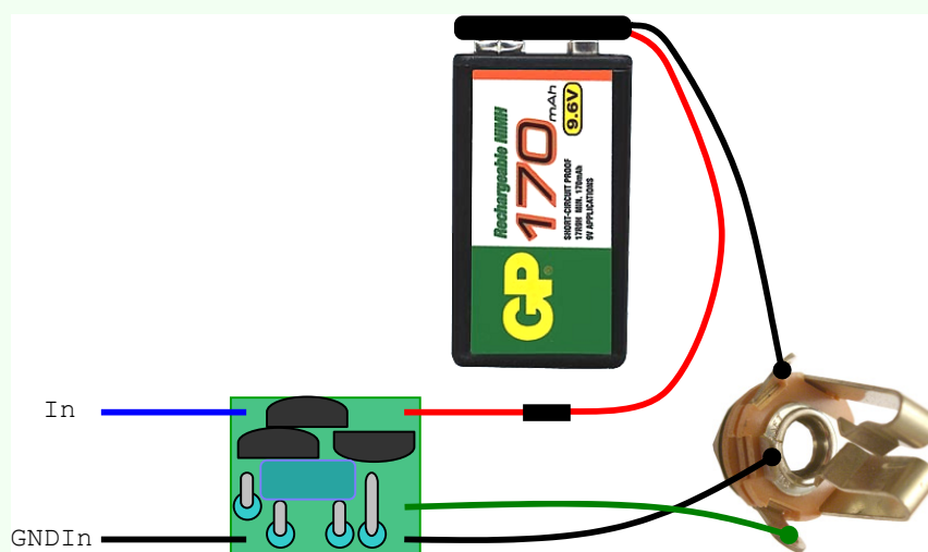
Abbildung 3-2: SB-1P-A1 direkt vor der Ausgangsbuchse
