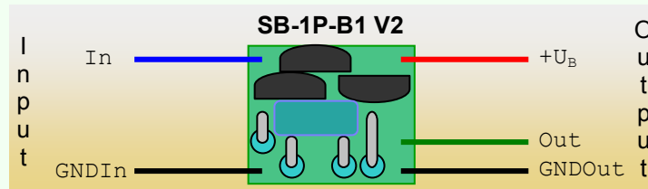
Abbildung 3-1: Die Platine des SB-1P-B1
