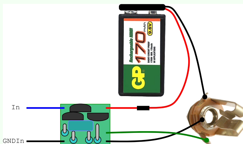
Abbildung 3-2: SB-1P-B1 direkt vor der Ausgangsbuchse
