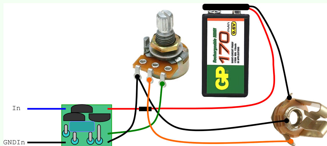
Abbildung 3-3: SB-1P-B1 mit Lautstärkeinsteller vor der Ausgangsbuchse
