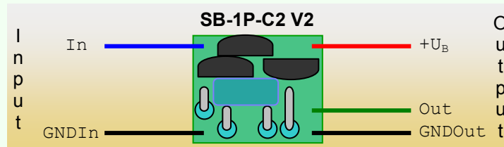
Abbildung 3-1: Die Platine des SB-1P-C2
