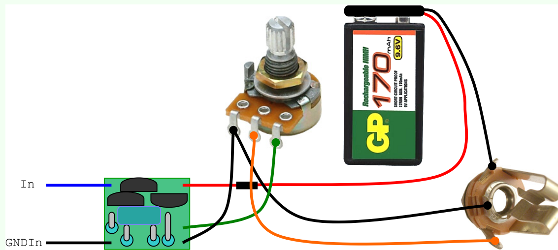
Abbildung 3-3: SB-1P-C2 mit Lautstärkeinsteller vor der Ausgangsbuchse
